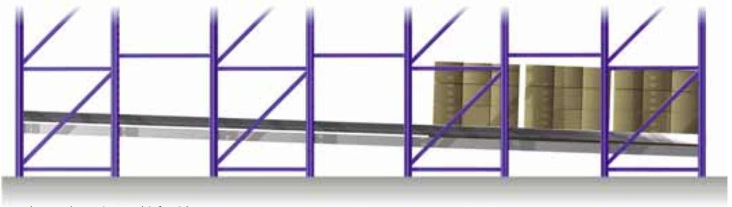
Ständeranordnung in Kanaltiefenrichtung
