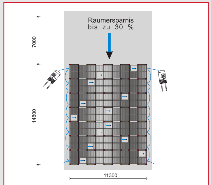
Fahrwege im META MULTILINE® S Durchlaufregal
