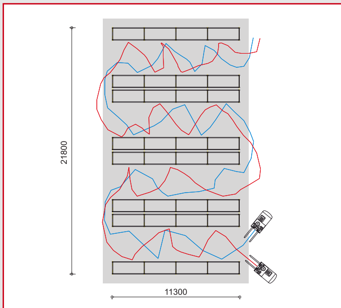
Fahrwege im konventionellen Palettenregal
