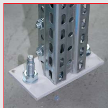
für die optimale Nivellierung der Regalanlage wird jeder Fuß höhenverstellbar ausgeführt
