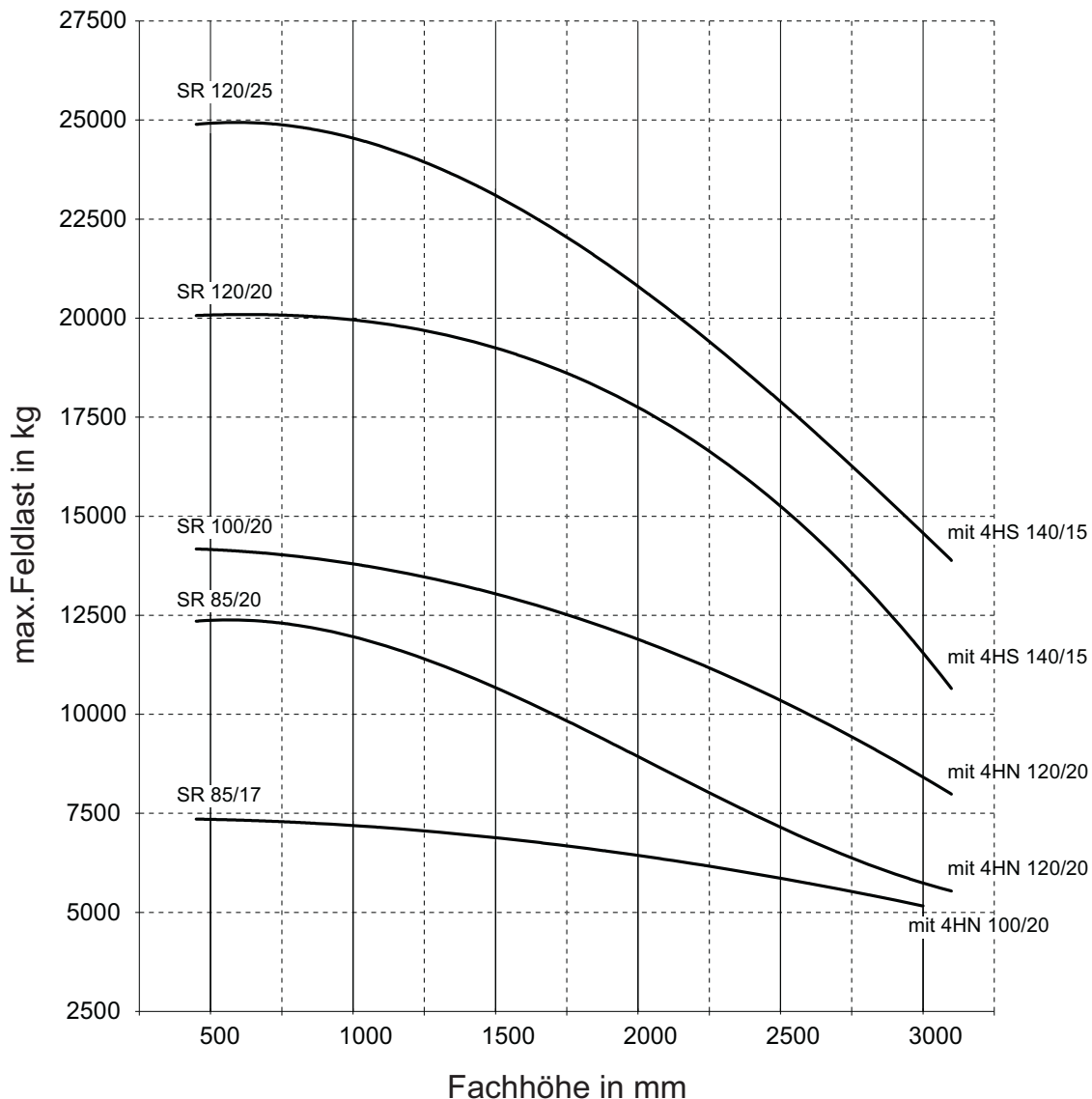
Feldlasten - Rahmenhöhe 8m - bei Fachweiten bis 2700mm
