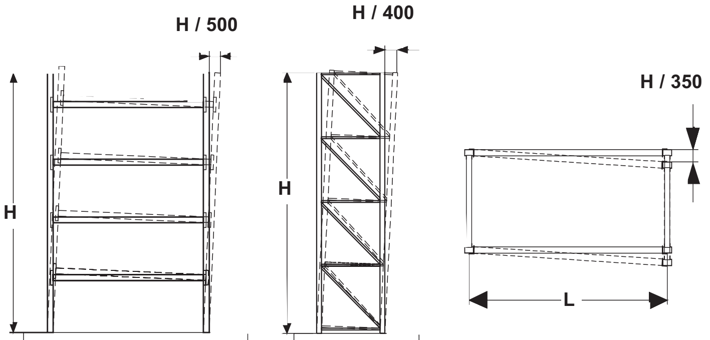
Regal-Längsrichtung longitudinal direction of racks sens longitudinal des rayonnages
